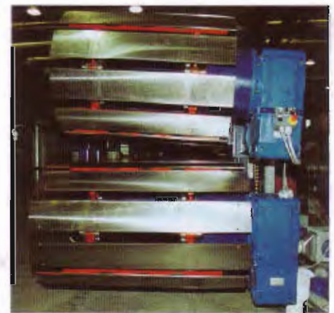
Конвейер для бумажных панелей, работающий со скоростью 60 м/мин, с наклоняющимся верхним ремнем
